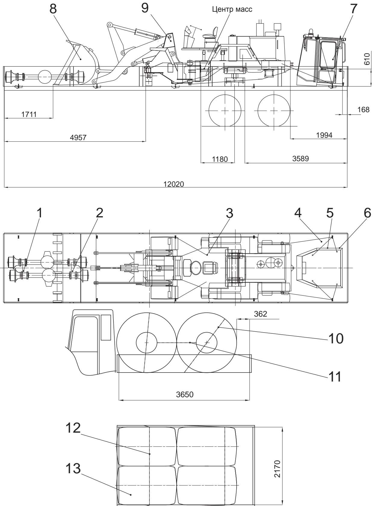
1 - 4 - растяжки; 5, 6, 10, 11, 12 - увязки; 7 - кабина; 8 - ковш; 9 - машина; 13 - колесо Рисунок 7.9 — Размещение и крепление на автотранспорте погрузчиков торфа АМКОДОР 342Р, АМКОДОР 342Р-01
