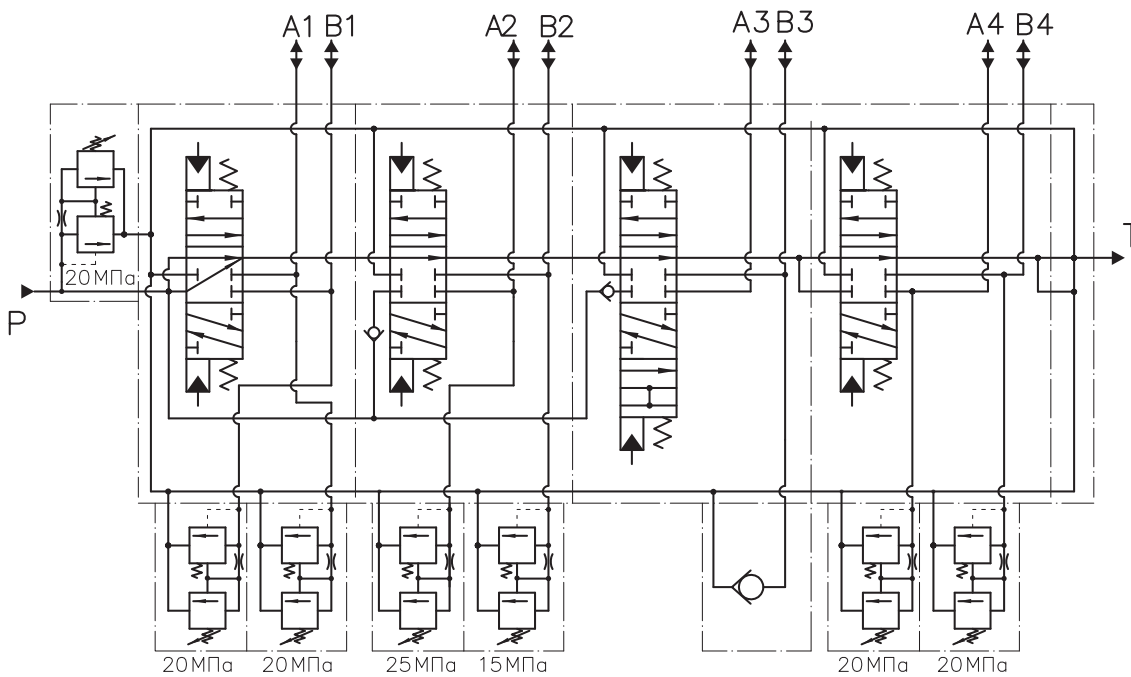
1 - клапан предохранительный; 6, 8 - клапаны реактивные; 7 - клапан обратный Рисунок 2.73 — Гидрораспределитель 4-секционный а) - основной вариант, б) - возможная комплектация распределителя производства ООО "САЛЕО"
